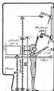
دوش، ملاحظات اندام‌سنجی کودکان
