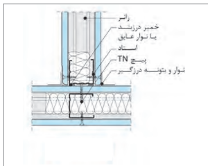
جزئیات پلان از اتصال دو دیوار دو لایه به یکدیگر (اتصال T)
