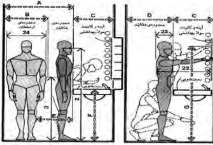
دست شویی، ملاحظات اندامسنجی مربوط به مردان
