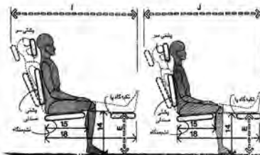
صنایعی عقب‌رو یا جانبی، افراد مذکر و مؤنث
